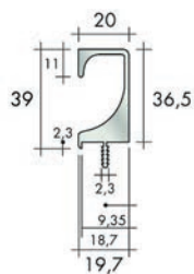
Profil poignée en aluminium type 900303
